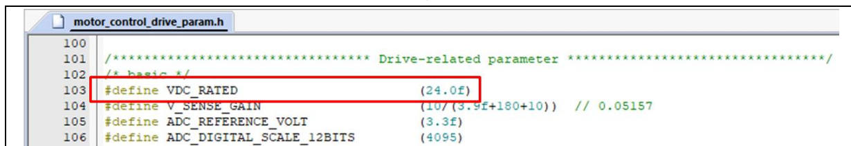
图 17. 电机额定电压
