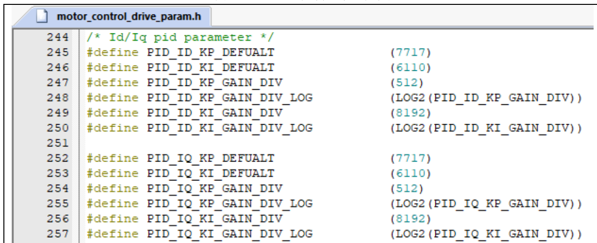
图 19. 电流 PI 控制参数宏定义
