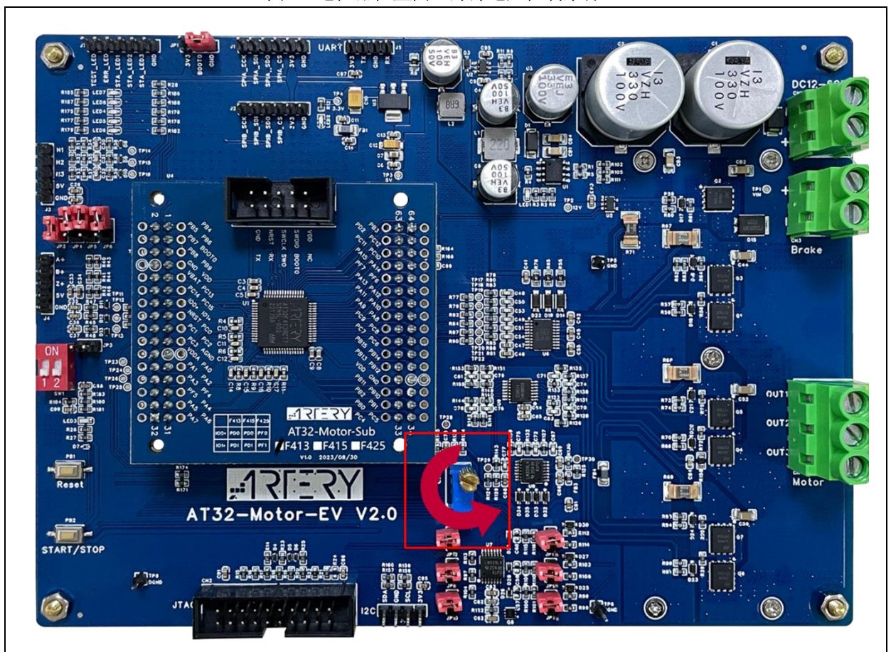
图 58. 电位器位置图（外部电压控制来源）
