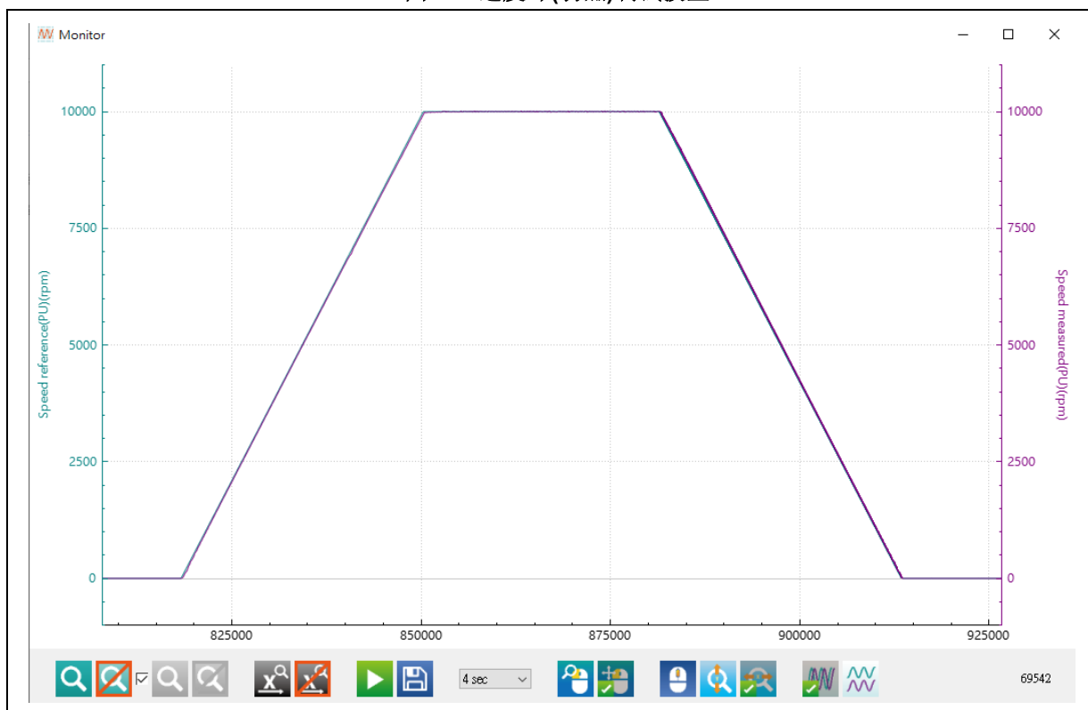
图 42. 速度环(弱磁)调试波形
