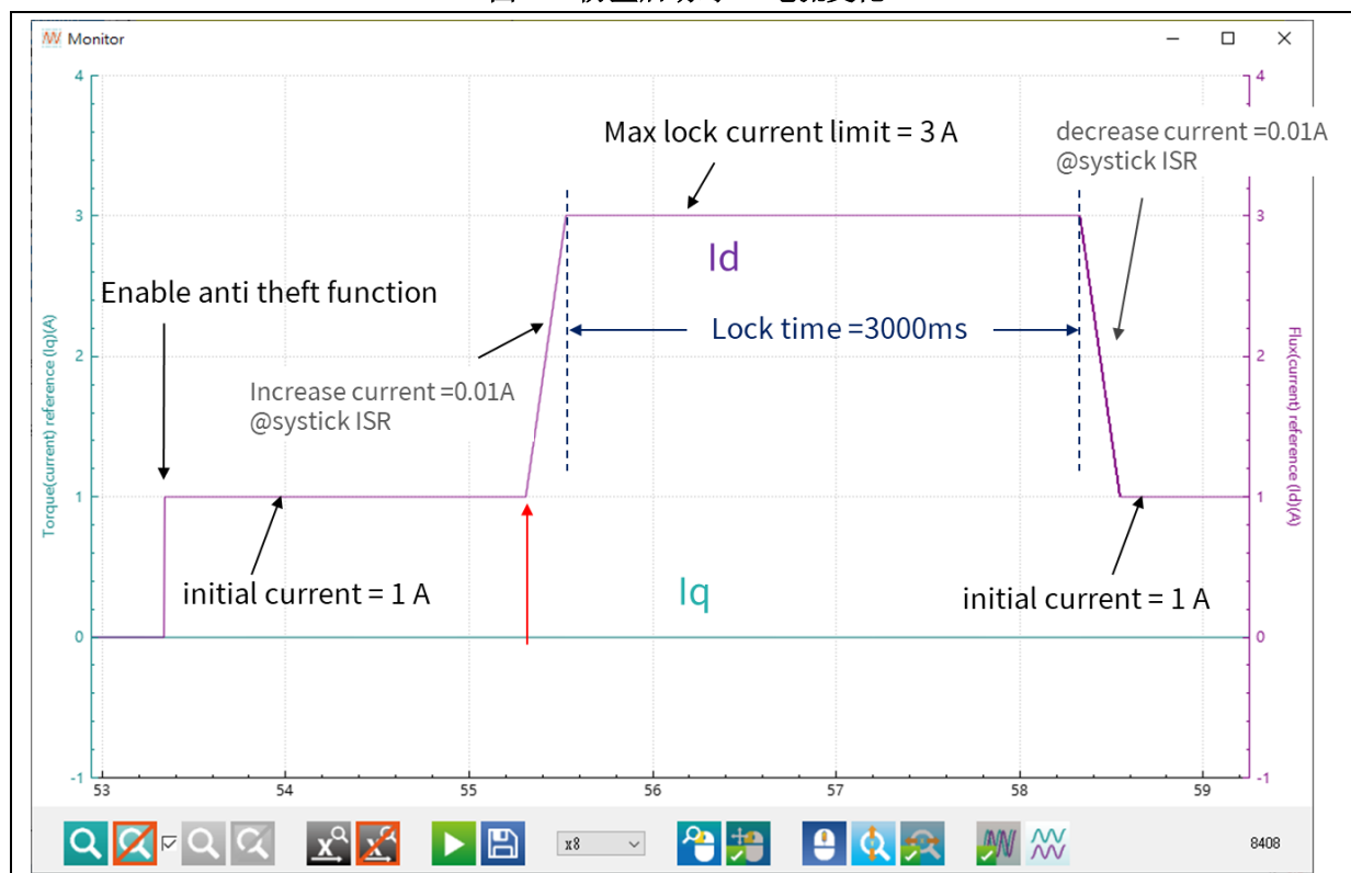
图 54. 防盗启动时 Id 电流变化
