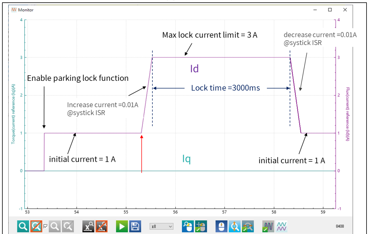
图 56. 驻车模式时 Id 电流变化
