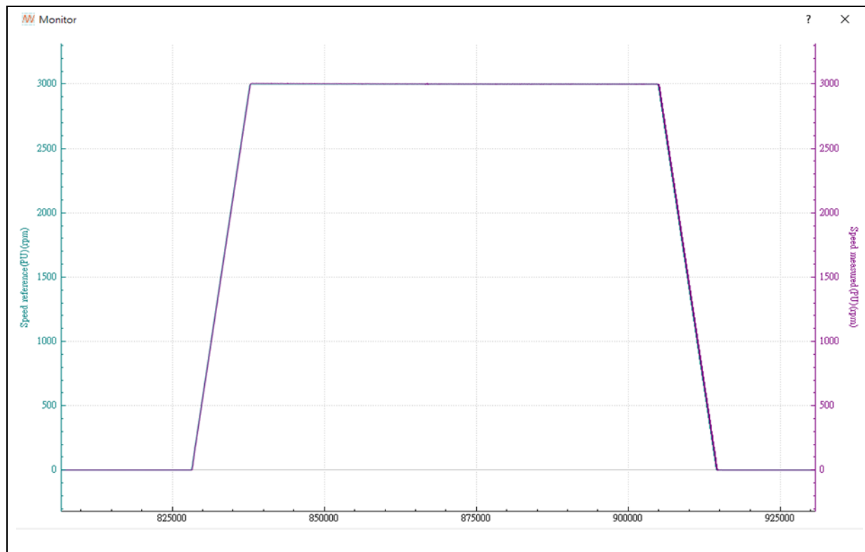
图 38. 速度环调试波形
