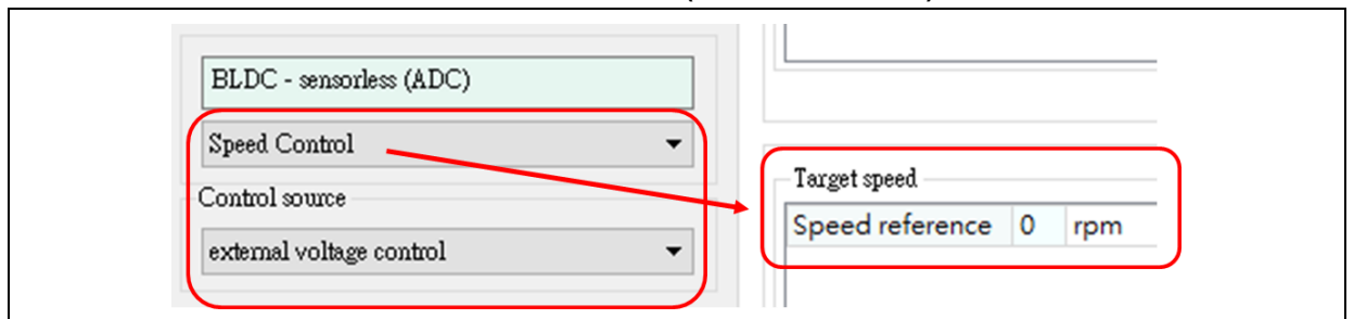
图 60. 速度控制模式(外部电压控制来源)
