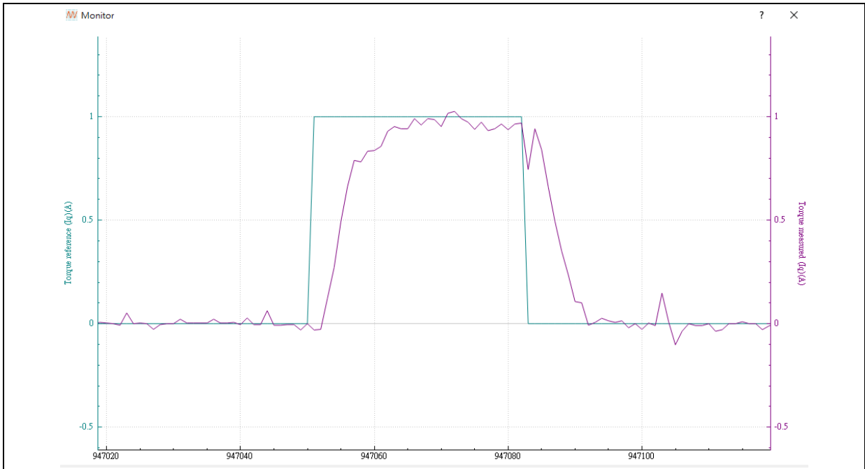
图 29. Q 轴电流环调试波形
