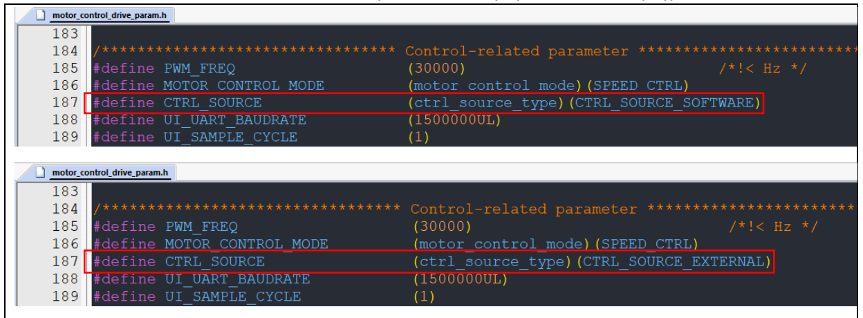
图 59. 控制来源定义值(软件控制来源(上)/外部电压控制(下))
