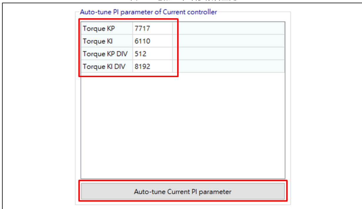
图 18. 电流 PI 控制参数自整定
