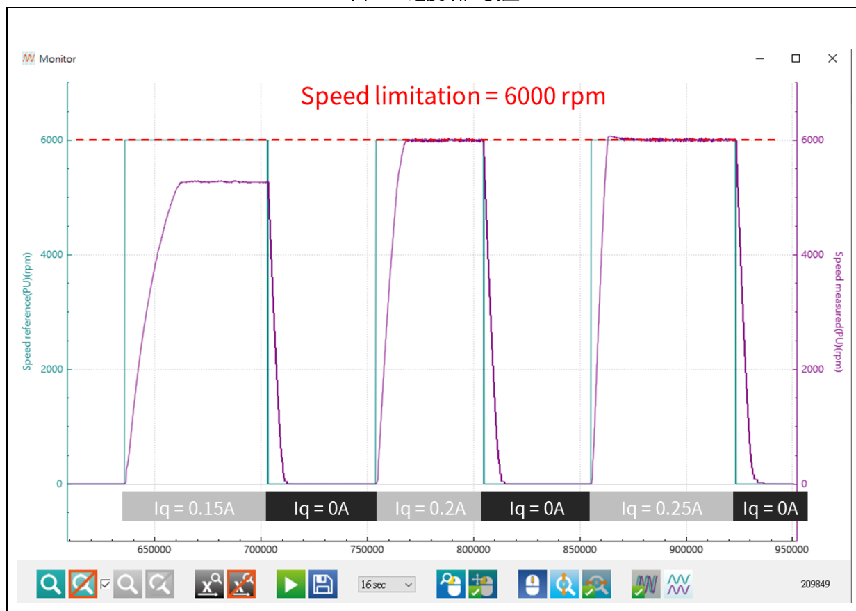
图 34. 速度响应波型
